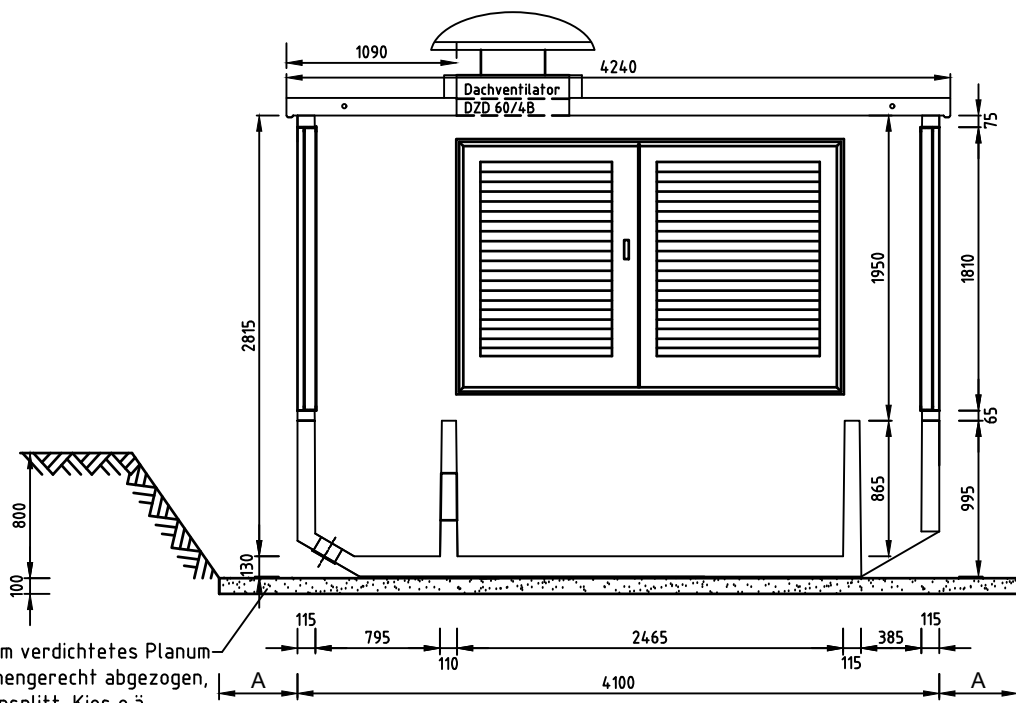
Schnitt B-B
